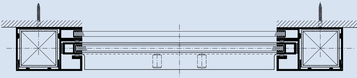
Befestigung nach hinten gegen Wand Fixation contre le mur
